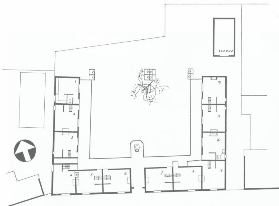
Plattegrond oude toestand.
